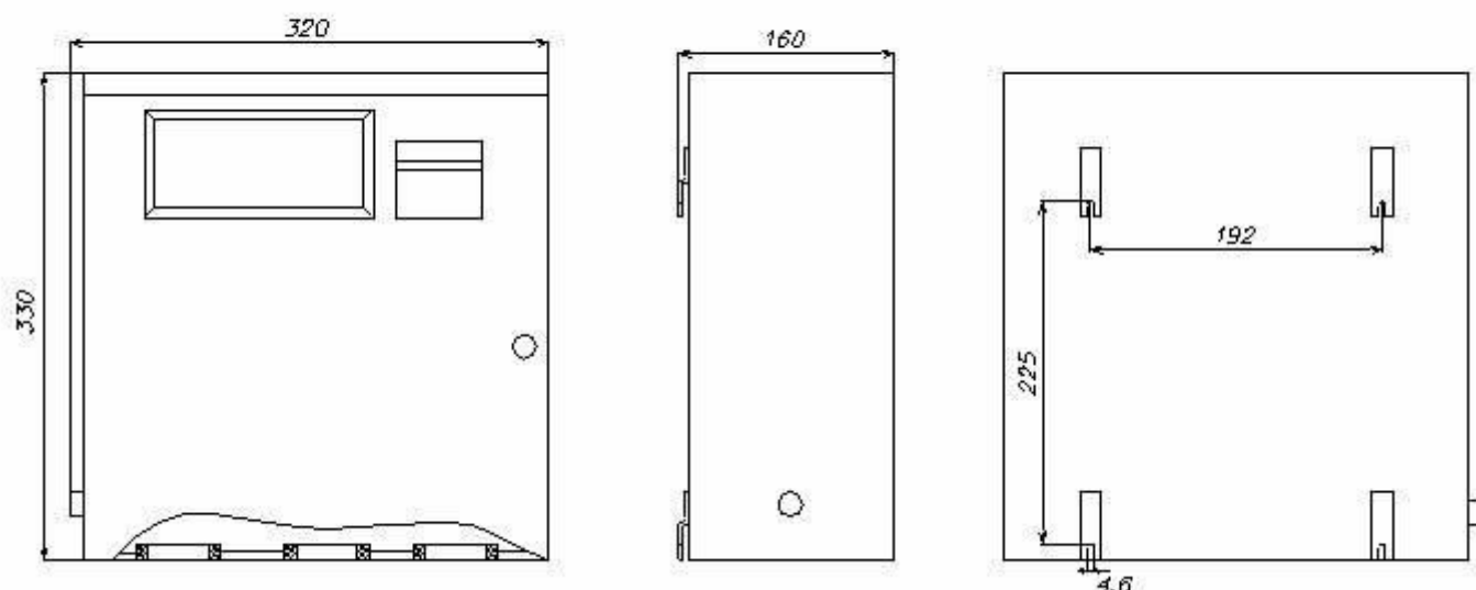
Габаритные и присоединительные размеры на станции управления СУЗ-10.
